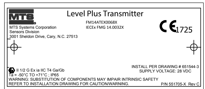
Fig. 57 : Étiquette ATEX/IECEx sécurité intrinsèque, Modbus ou DDA, boîtier à cavité simple ou double
