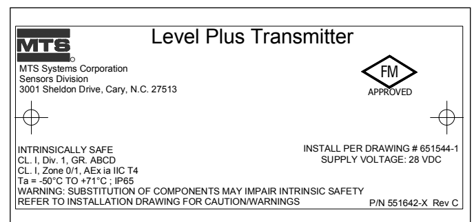
Fig. 21 : Étiquette FM sécurité intrinsèque, HART®, boîtier à cavité simple ou double
