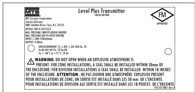
Fig. 46 : Antidéflagrant, étiquette FMC, HART®, option de boîtier G, H ou L
