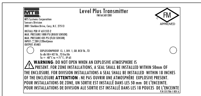
Fig. 44 : Antidéflagrant, étiquette FMC, Modbus ou DDA, option de boîtier Option G, H ou L
