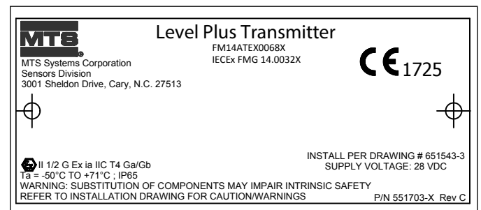
Fig. 56 : Étiquette ATEX/IECEx sécurité intrinsèque, Modbus ou DDA, boîtier à cavité simple ou double
