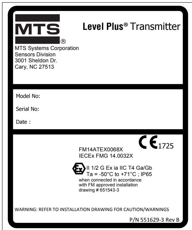
Fig. 54 : Étiquette FMC sécurité intrinsèque, Modbus ou DDA, boîtier NEMA
