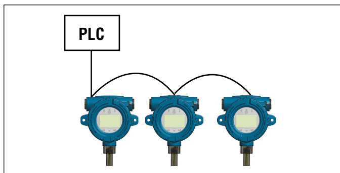
Fig. 13: Topología de cadena tipo margarita
