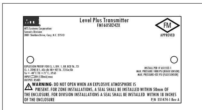
Fig. 23: Resistente a explosiones, etiqueta FM, Modbus o DDA, opción de carcasa G, H o L
