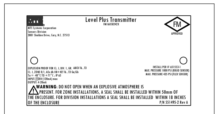
Fig. 26: Resistente a explosiones, etiqueta FM, HART®, opción de carcasa D, E
