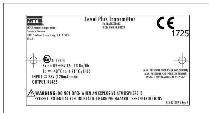
Fig. 59: Ignífugo, etiqueta ATEX/IECEX, Modbus o DDA, opción de carcasa D, E, G, H o L
