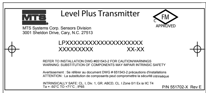
Fig. 33: Etiqueta FMC de seguridad intrínseca, Modbus y DDA, carcasa con cavidad individual y doble
