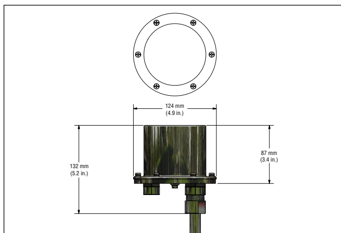
Fig. 1: Carcasa de acero inoxidable Tipo NEMA 4X 316L
