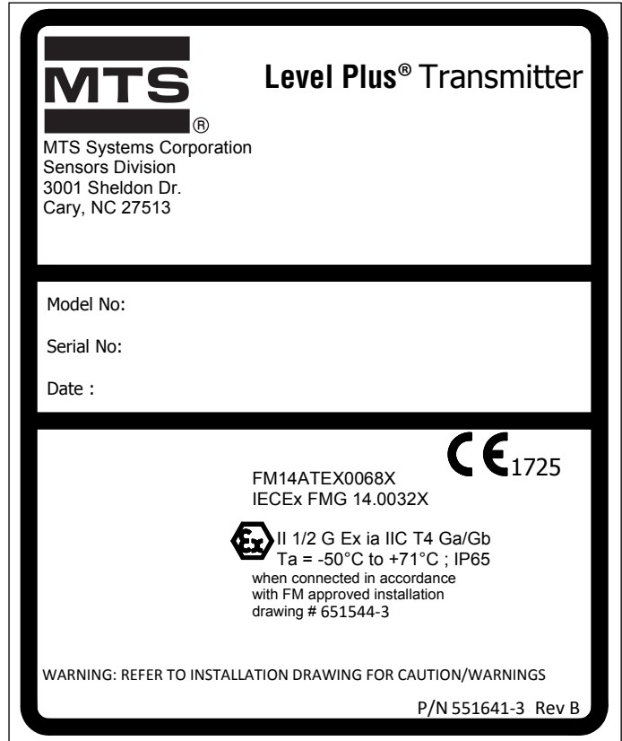
Fig. 52: Etiqueta ATEX/IECEx de seguridad intrínseca, Modbus y DDA, carcasa NEMA
