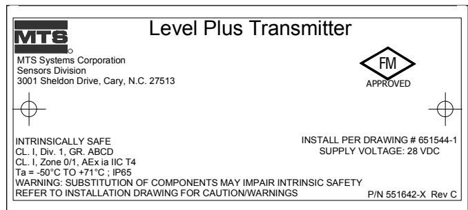
Fig. 18: Etiqueta FM de seguridad intrínseca, HART®, carcasa con cavidad individual o doble
