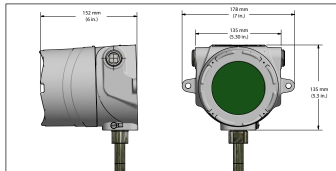
Fig. 4: Carcasa de acero inoxidable con cavidad individual
