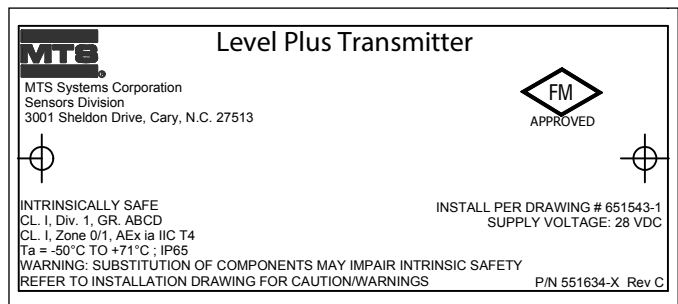
Fig. 17: Etiqueta FM de seguridad intrínseca, Modbus o DDA, carcasa con cavidad individual o doble
