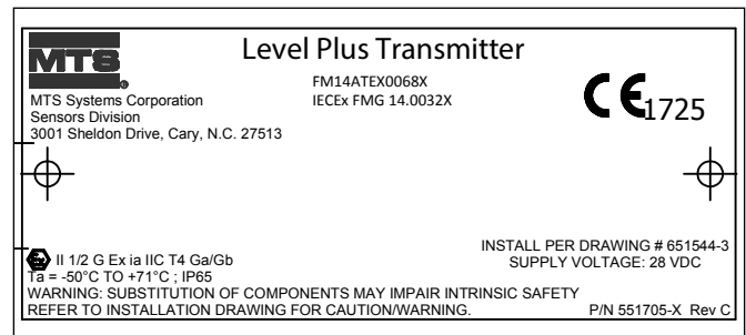
Fig. 54: Etiqueta ATEX/IECEx de seguridad intrínseca, Modbus y DDA, carcasa con cavidad individual y doble
