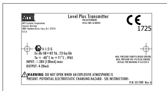
Fig. 60: Ignífugo, etiqueta ATEX/IECEX, HART®, opción de carcasa D, E, G, H o L
