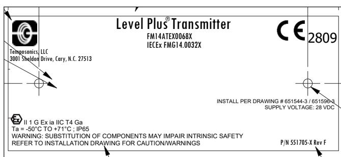
Fig. 54: Etichetta di Sicurezza intrinseca ATEX/IECEX, Modbus e DDA, custodia con intercapedine singola e doppia
