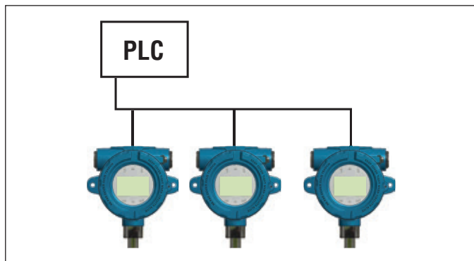
Fig. 11: Topologia bus con spur
