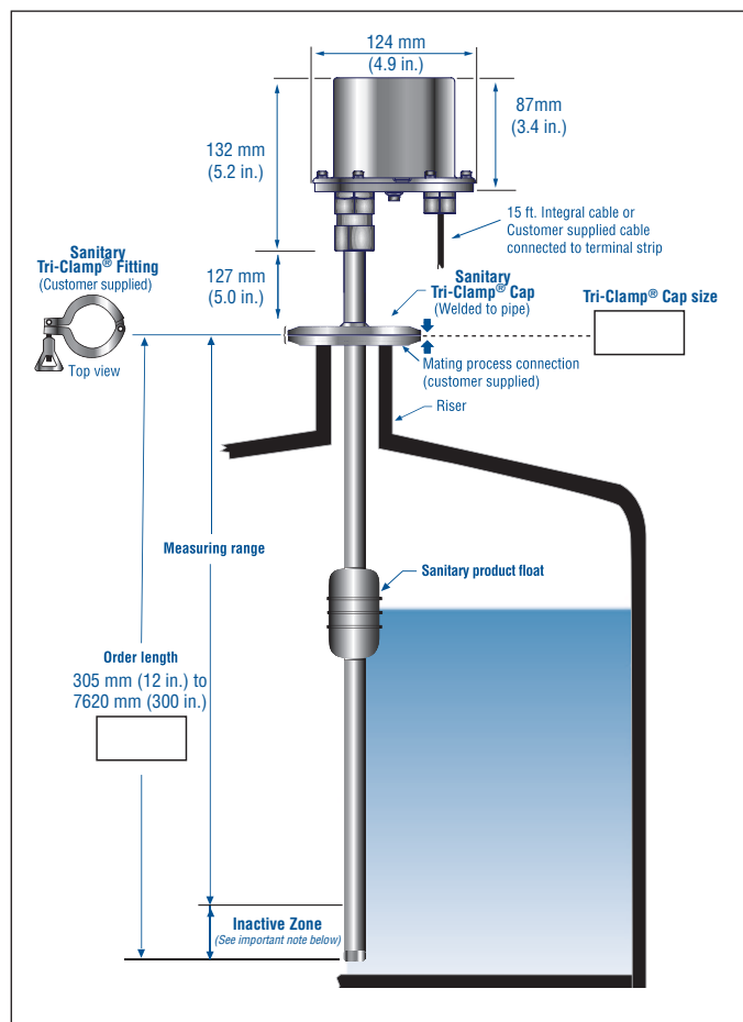
Fig. 9: Montaggio del tubo con Tri-Clamp
