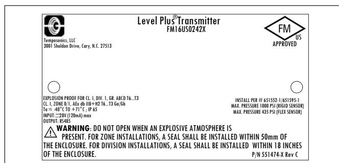
Fig. 24: Antideflagrante, etichetta FM, Modbus o DDA, opzione custodia D, E
