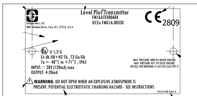
Fig. 60: Ignifugo, etichetta ATEX e IECEX, HART®, custodia opzione D, E, G, H o L
