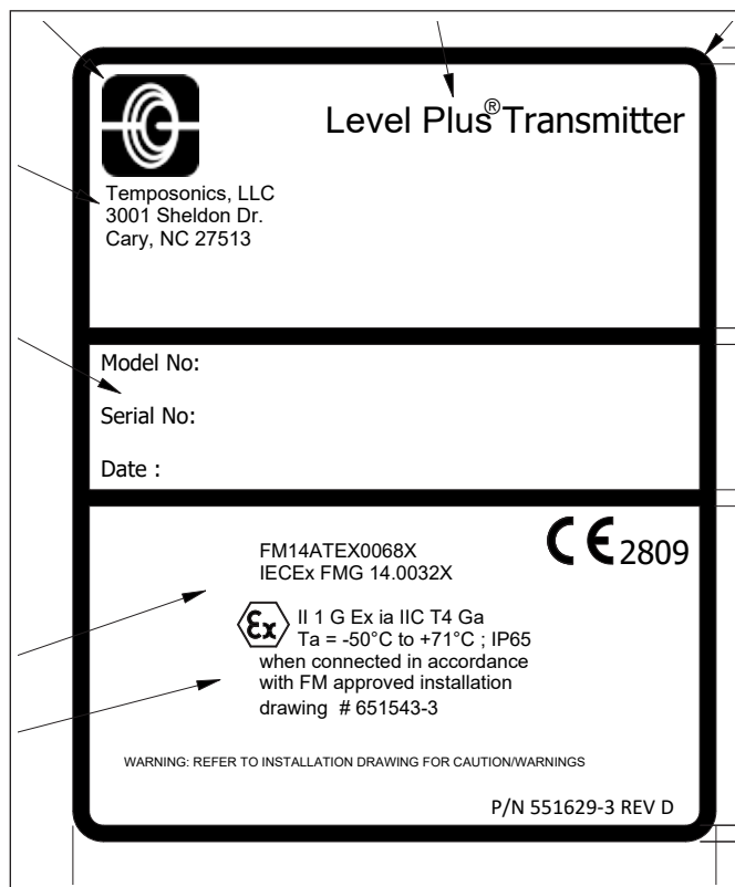
Abb. 51: FMC-Kennzeichnung Eigensicherheit, Modbus und DDA, NEMA-Gehäuse
