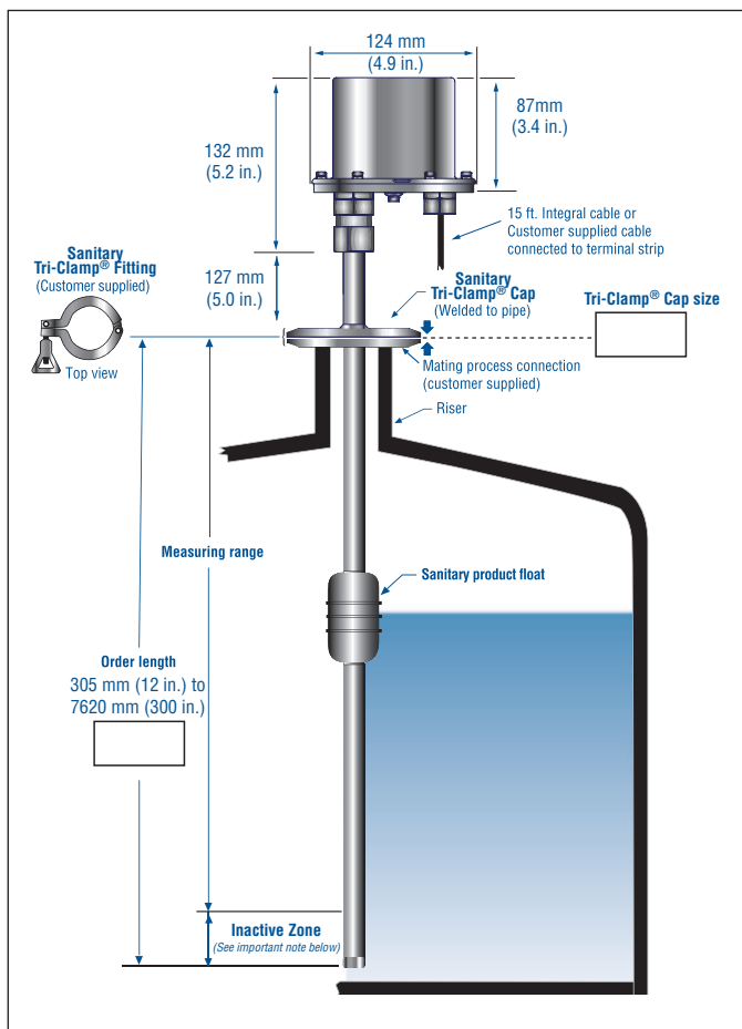
Abb. 9: Montage Tri-Clamp-Anschluss für Rohr
