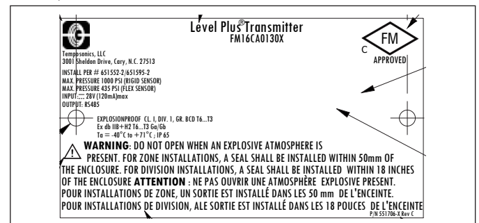
Abb. 42: Explosionsgeschützt, FMC-Kennzeichnung, Modbus oder DDA, Gehäuseoption D, E
