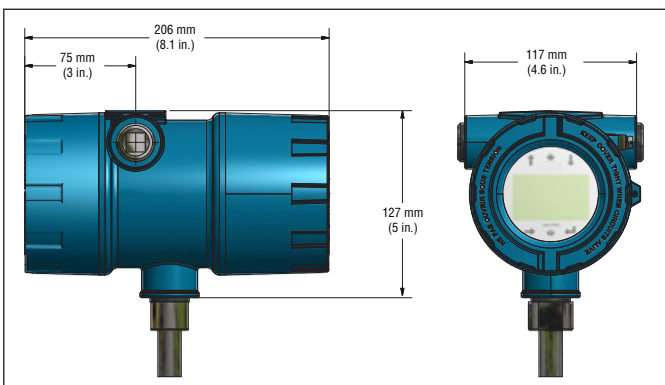
Abb. 3: Duales Hohlraumgehäuse
