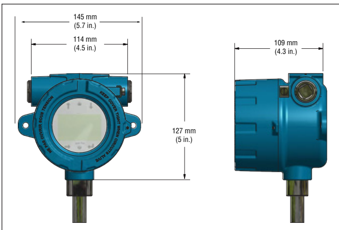
Abb. 2: Einfaches Hohlraumgehäuse
