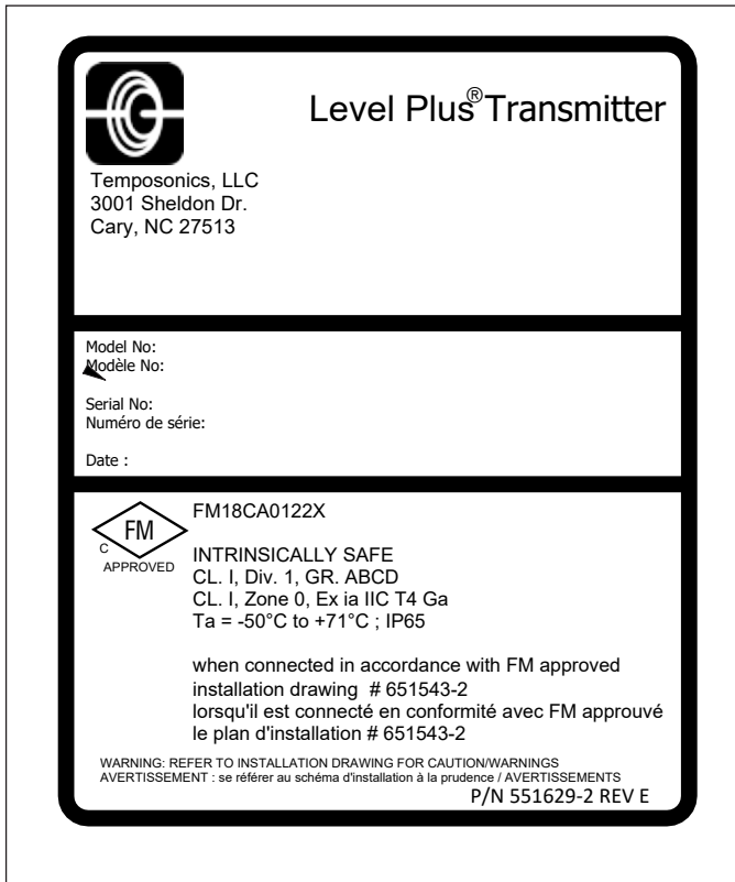
Abb. 31: FMC-Kennzeichnung Eigensicherheit, Modbus und DDA, NEMA-Gehäuse
