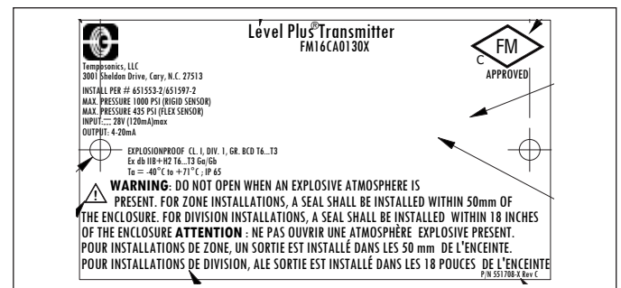
Abb. 44: Explosionsgeschützt, FMC-Kennzeichnung, HART®, Gehäuseoption D, E
