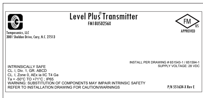
Abb. 17: FM-Kennzeichnung Eigensicherheit, Modbus oder DDA, einfaches oder duales Hohlraumgehäuse
