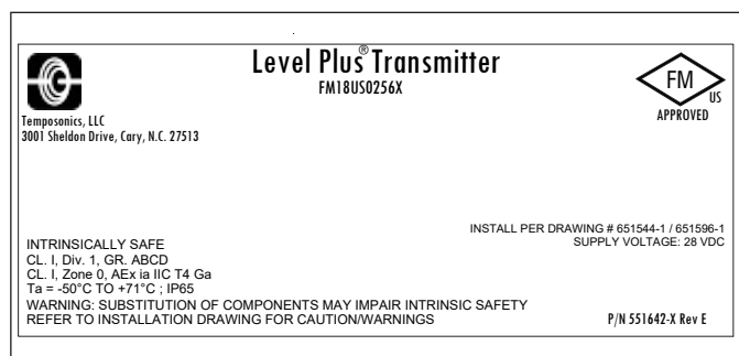
Abb. 18: FM-Kennzeichnung Eigensicherheit, HART®, einfaches oder duales Hohlraumgehäuse
