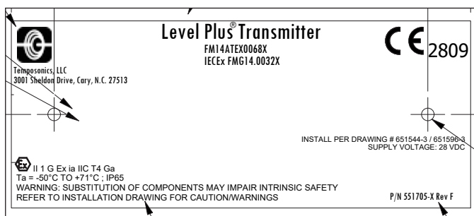
Abb. 54: ATEX/IECEx-Kennzeichnung Eigensicherheit, Modbus und DDA, einzelnes oder duales Hohlraumgehäuse
