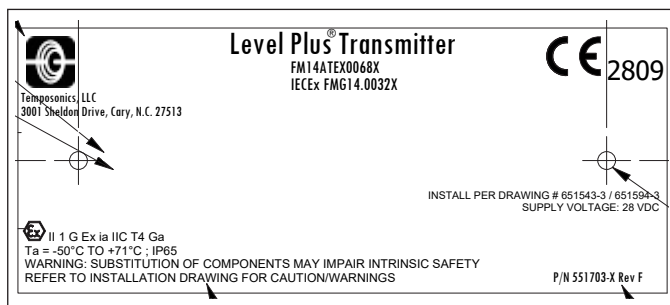
Abb. 53: ATEX/IECEx-Kennzeichnung Eigensicherheit, Modbus und DDA, einzelnes oder duales Hohlraumgehäuse
