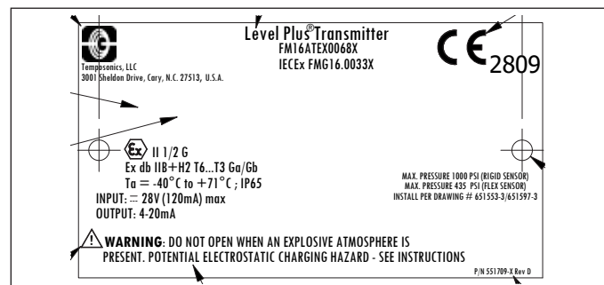
Abb. 60: Druckfest, ATEX- und IECEx-Kennzeichnung, HART®, Gehäuseoption D, E, G, H oder L
