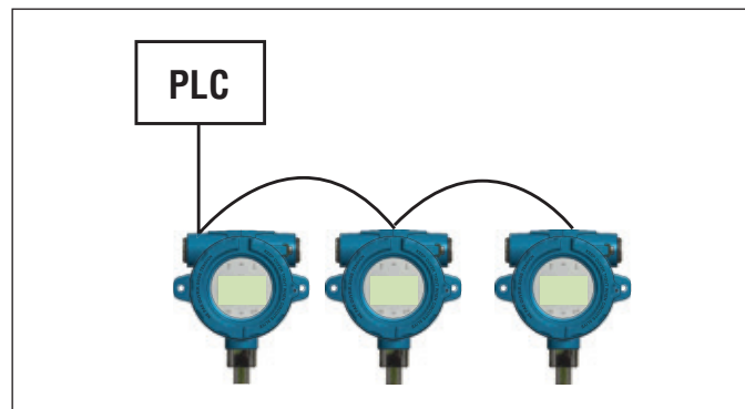
Abb. 13: Daisy-Chain-Topologie
