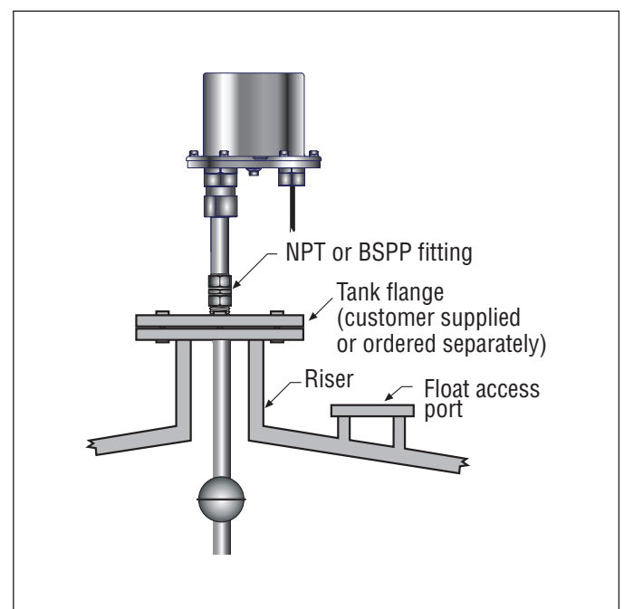
Abb. 8: Montage mit Gewindeflansch für flexiblen Schlauch
