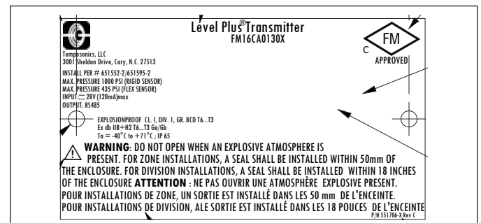
Abb. 43: Explosionsgeschützt, FMC-Kennzeichnung, HART®, Gehäuseoption G, H oder L
