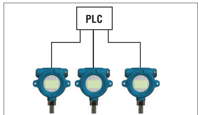
Abb. 10: Punkt-zu-Punkt-Topologie
