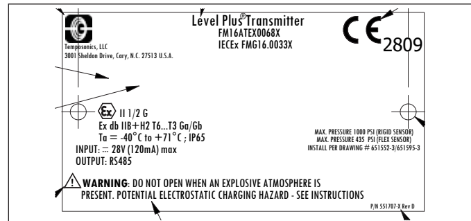
Abb. 59: Druckfest, ATEX- und IECEx-Kennzeichnung, Modbus oder DDA, Gehäuseoption D, E, G, H oder L
