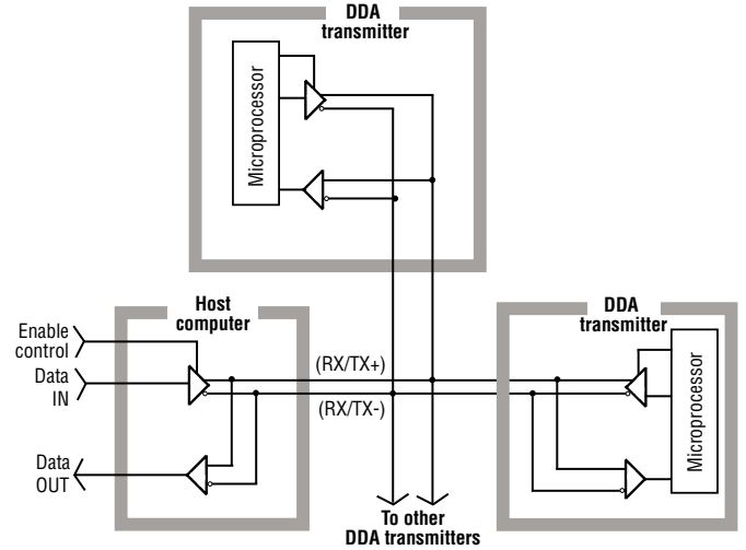
그림 4: RS-485 멀티 드롭 예시
