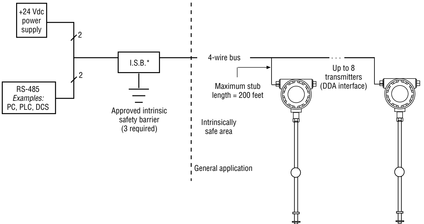
그림 3: 일반적인 전기 연결 - 본질 안전 시스템
